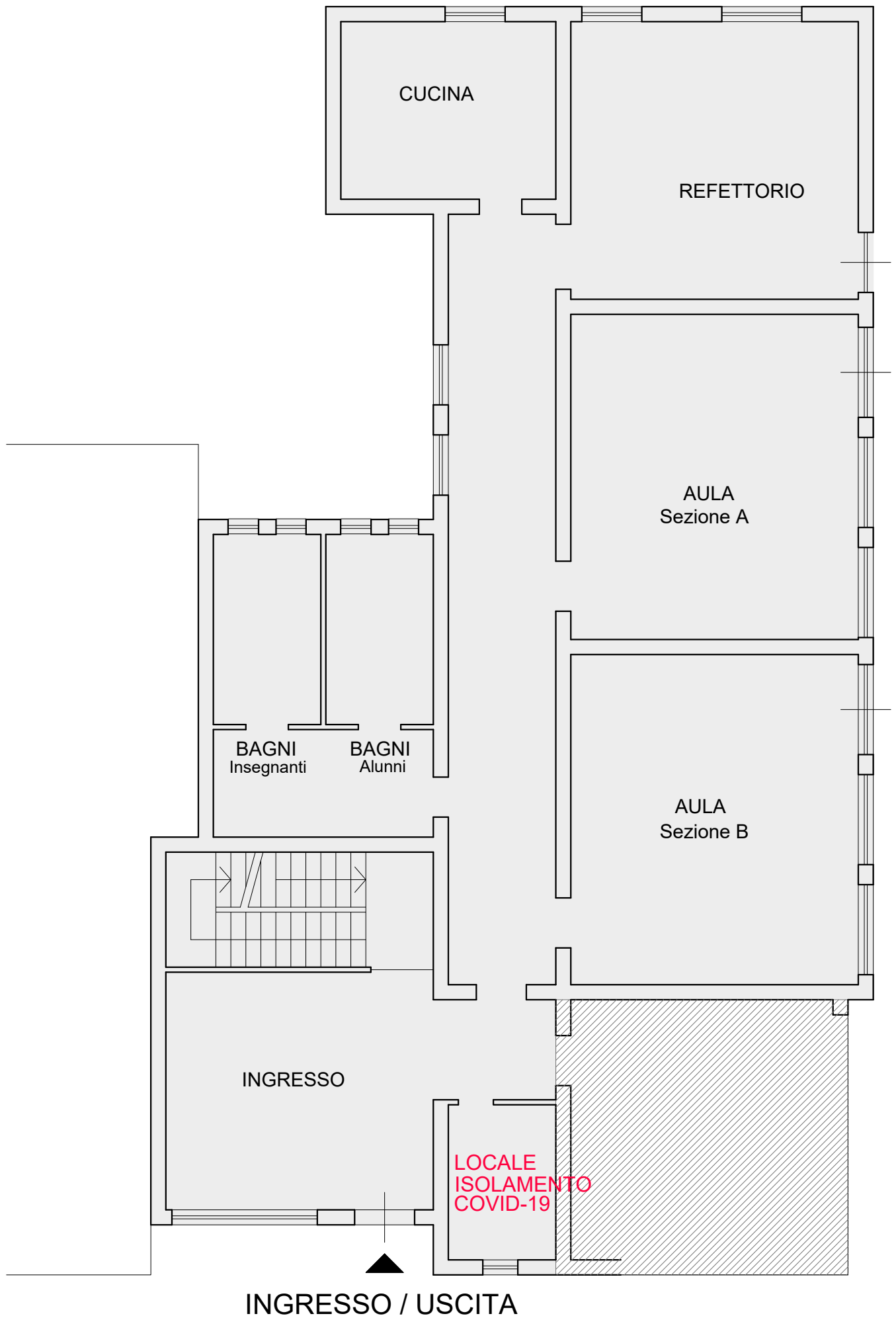
SCUOLA DELL'INFANZIA S. MICHELE PIANTA PIANO TERRA - scala 1:100
